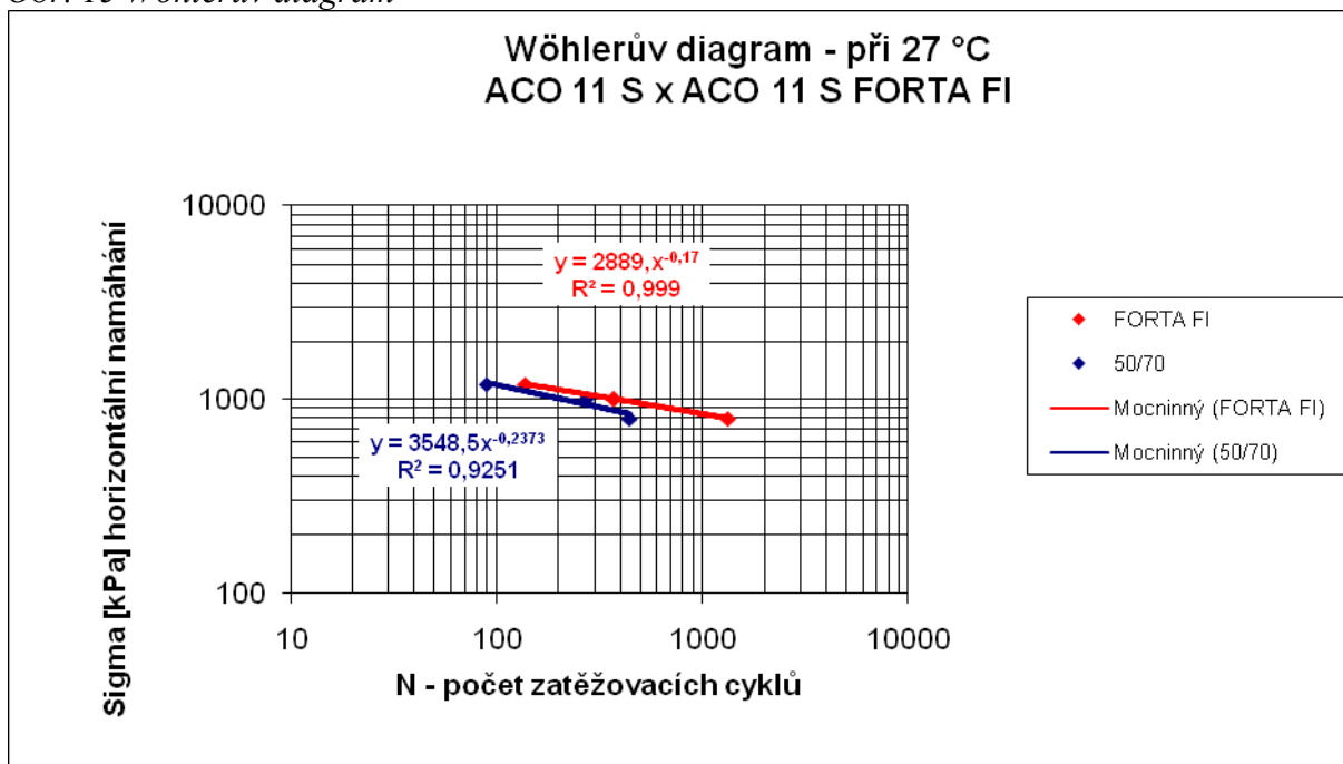
Obr. 15 Wöhlerův diagram
